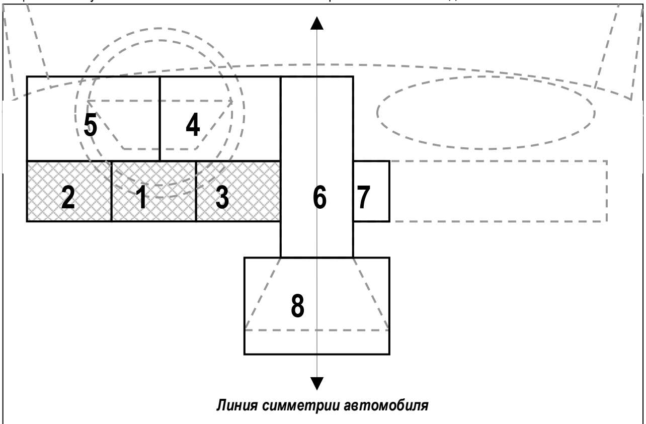
Места расположения колодки OBD-II
