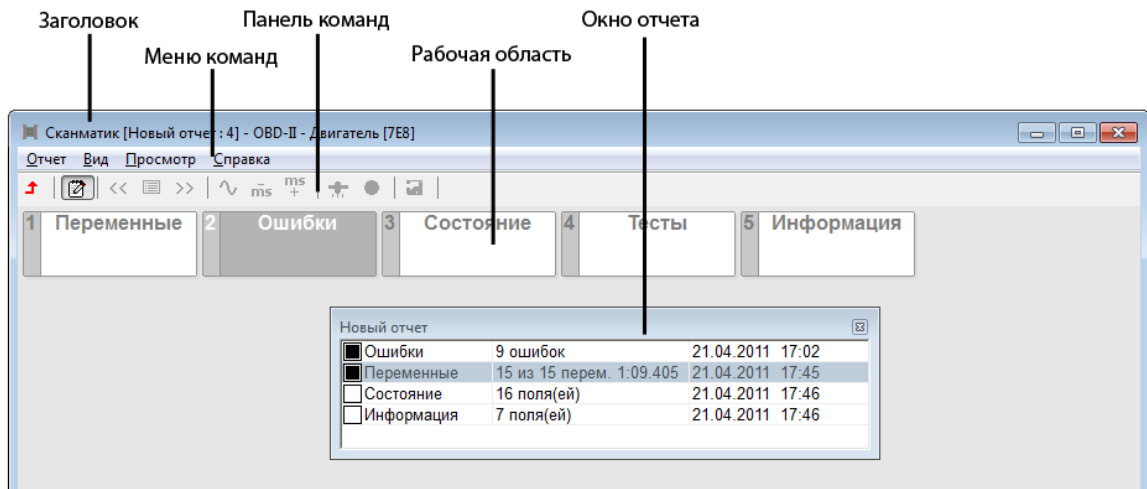
Интерфейс программы
