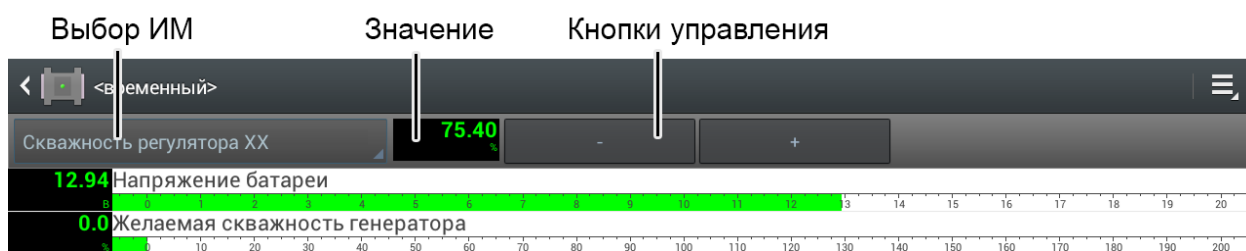
Панель управления ИМ
