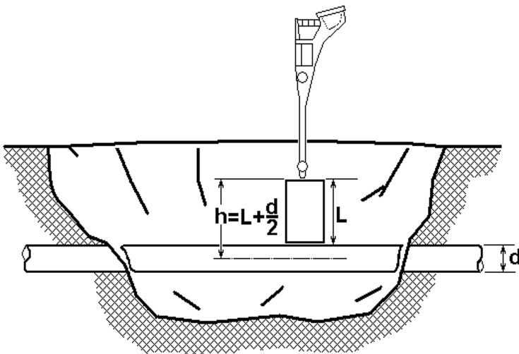
Калибровка на реальном трубопроводе
