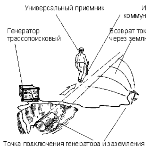
Общая схема поиска
